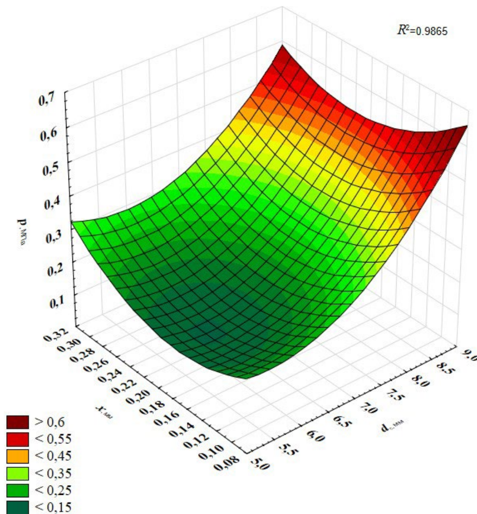
Рисунок 4.3 – График зависимости влияния глубины внедрения винта рассекателя в струю и диаметра сопла на интенсивность подачи воды
