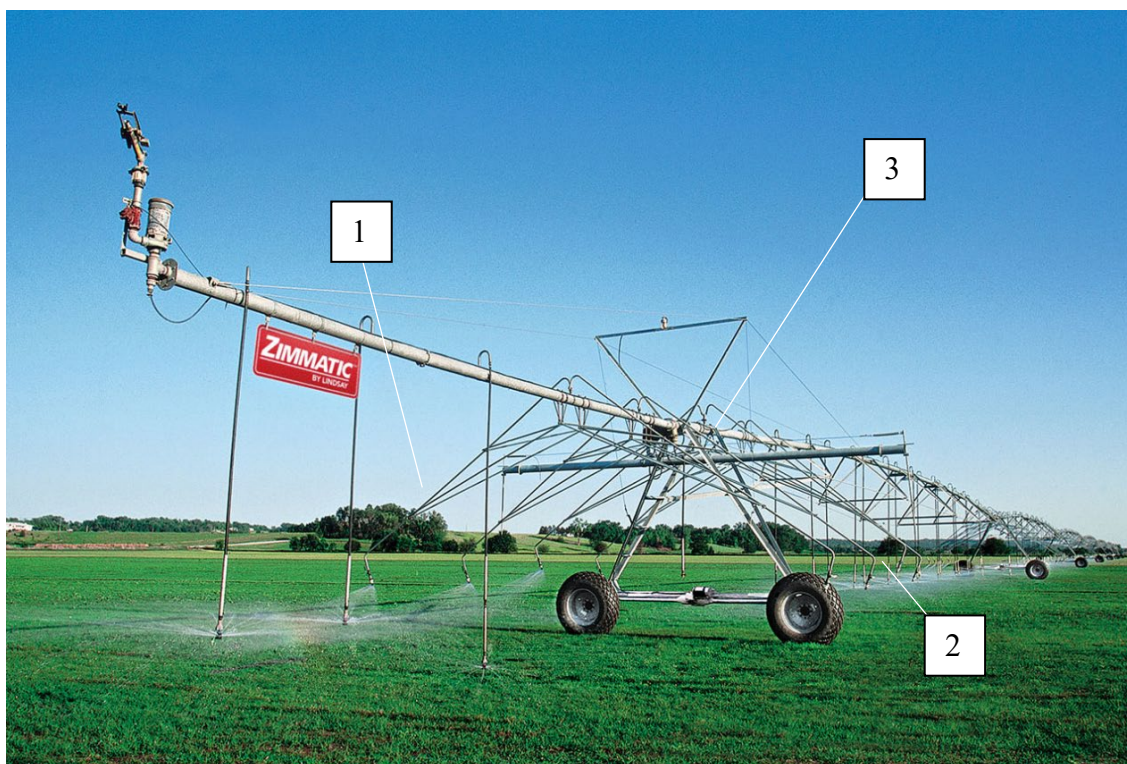
1 – открьлок; 2 – дождевальные насадки; 3 – центральный трубопровод Рисунок 1.17 – Вынос дождевальных аппаратов на ДМ «Zimmatic»
