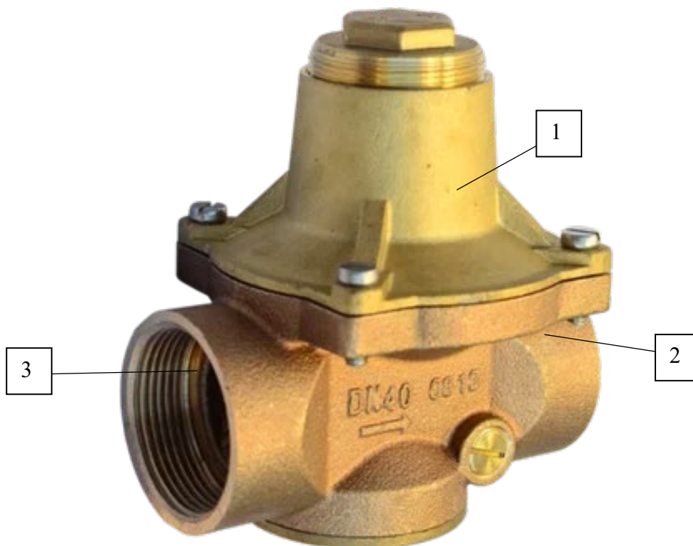
Рисунок 1.23 – Общий вид регулятора давления NELSON с дождевальной насадкой
