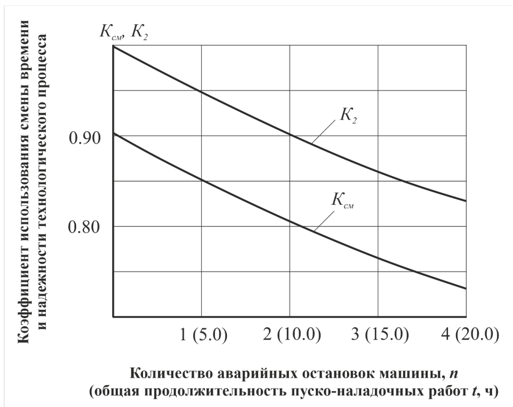
Рисунок 2.3 – Зависимость коэффициента использования времени смены K_{CM} от количества аварийных остановок дождевальной машины
