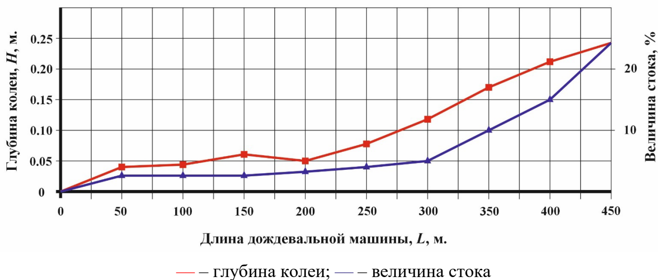
Рисунок 1.12 – Зависимость глубины колеи ходовых систем от величины стока по длине дождевальная машины
