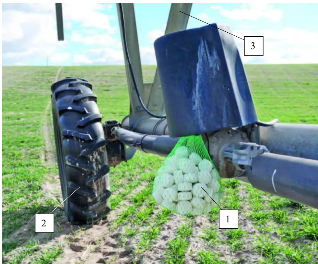
Рисунок 1.14 – Использование абсорбента на дождевальная машине
