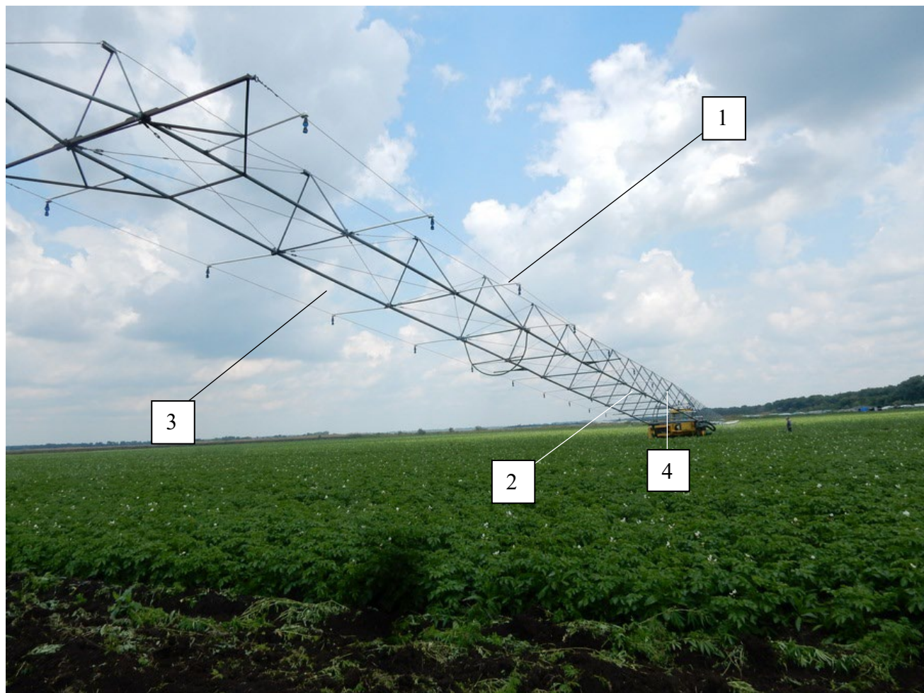
Рисунок 1.3 – Дальнеструйная дождевальная машина ДДА-100МА
