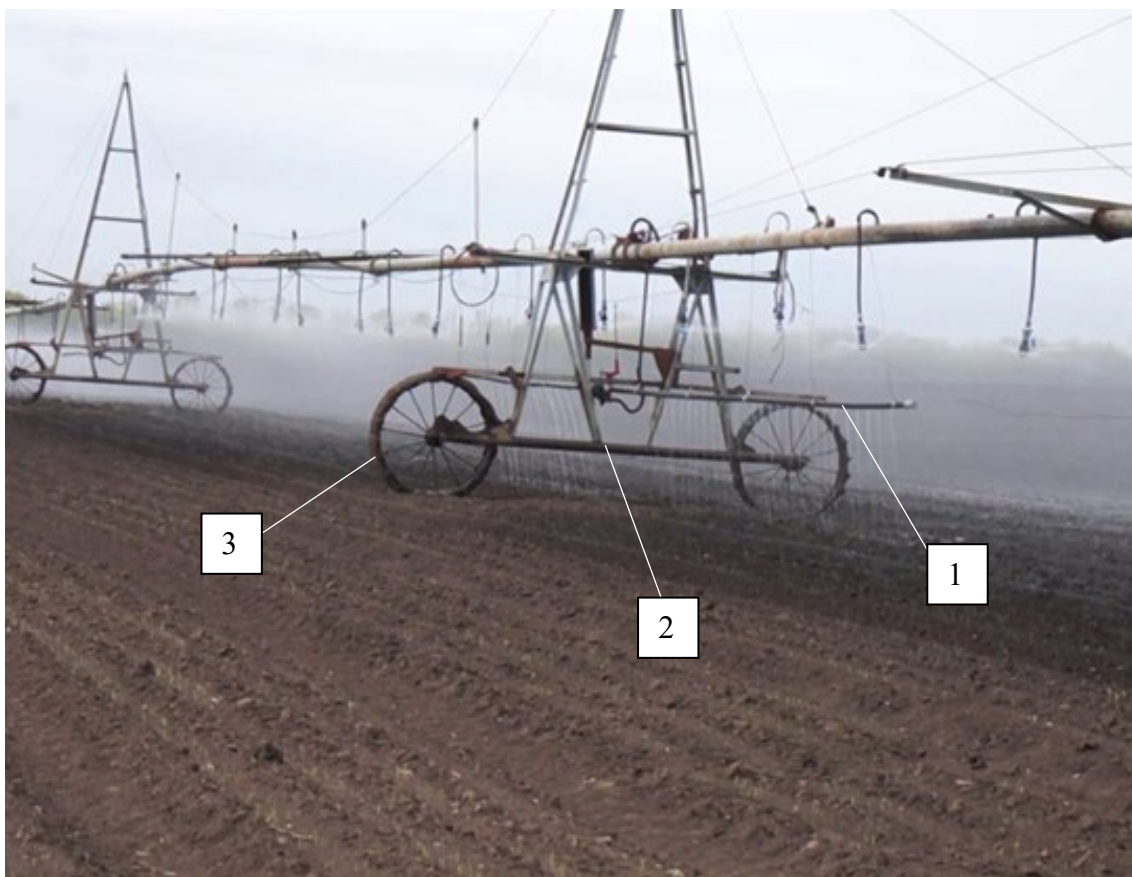
1 – модернизированный слив; 2 – самоходная тележка; 3 – жесткое колесо Рисунок 1.18 – Система слива отработанной воды гидроцилиндрами ДМ «Фрегат»
