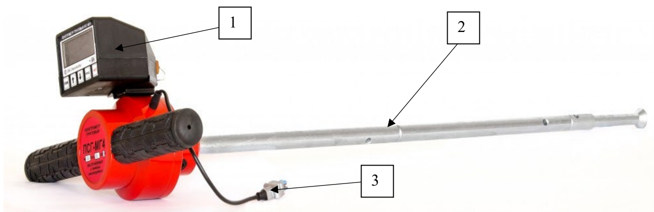
1 – прибор; 2 – рабочий наконечник; 3 – USB кабель связи с ПК
