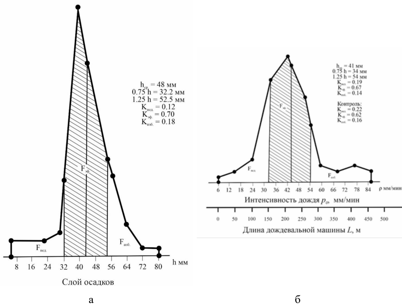
Рисунок 4.9 – Частотный график равномерности распределения слоя воды по длине дождевальной машины
