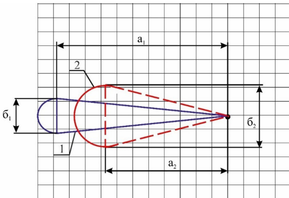
Рисунок 2.9 – Площадь полива дождевальным аппаратом «Фрегат №3»
