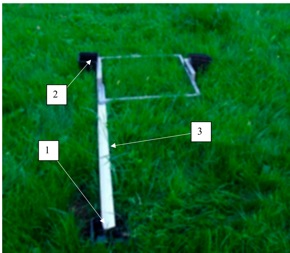
1 – дождемер; 2 – стоковая рамка; 3 – сливная трубка
