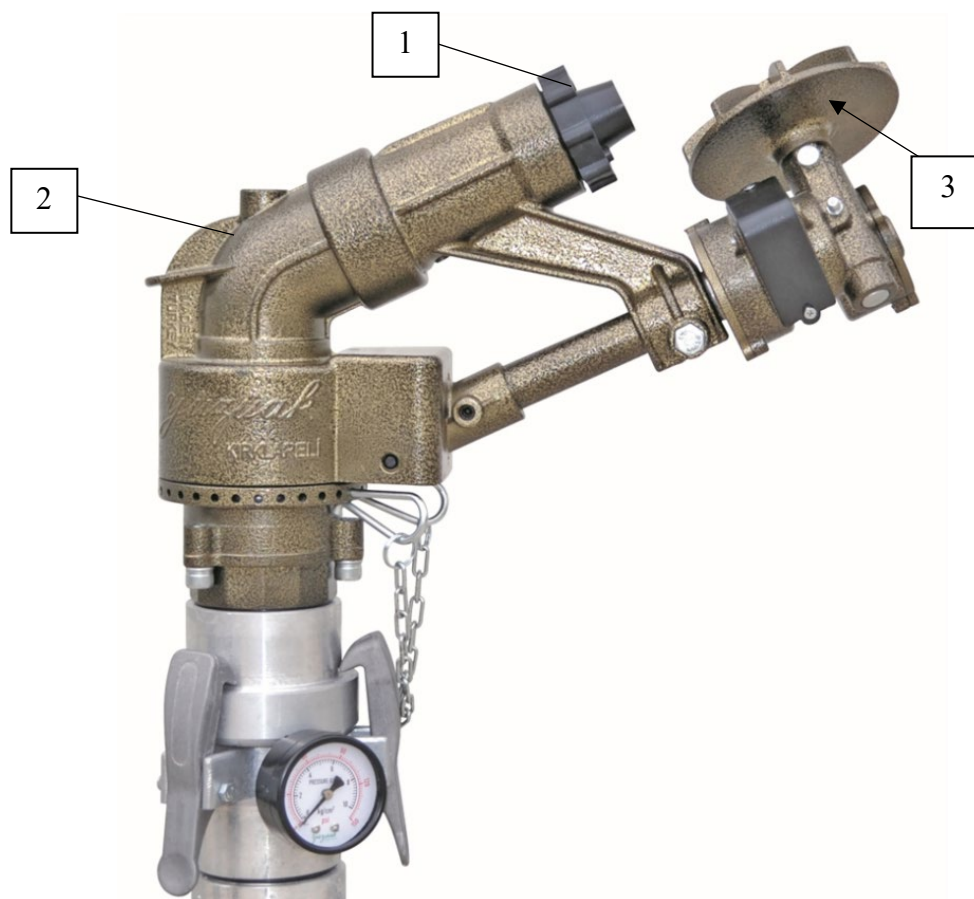
1 – сопло; 2 – ствол аппарата; 3 – турбинный рассекатель
