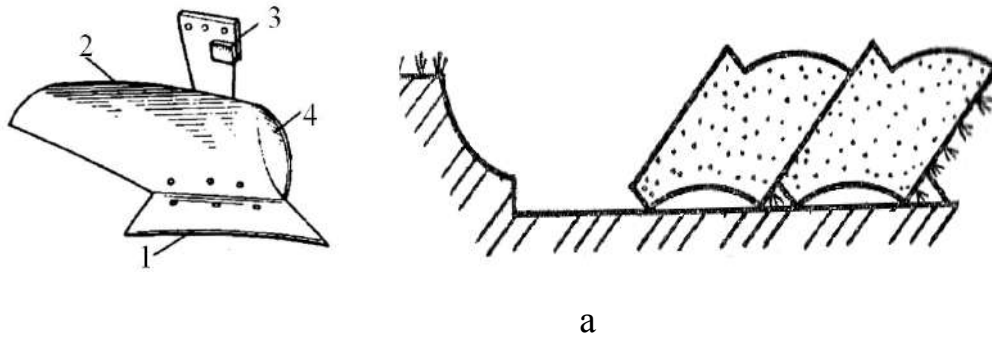
Рисунок 1.6.- Корпус плуга с ромбовидными отвалами 1 – лемех; 2 – отвал; 3 – стойка; 4 – лемех боковой. а - схема поперечного разреза пластов вспаханных ромбовидными корпусами
