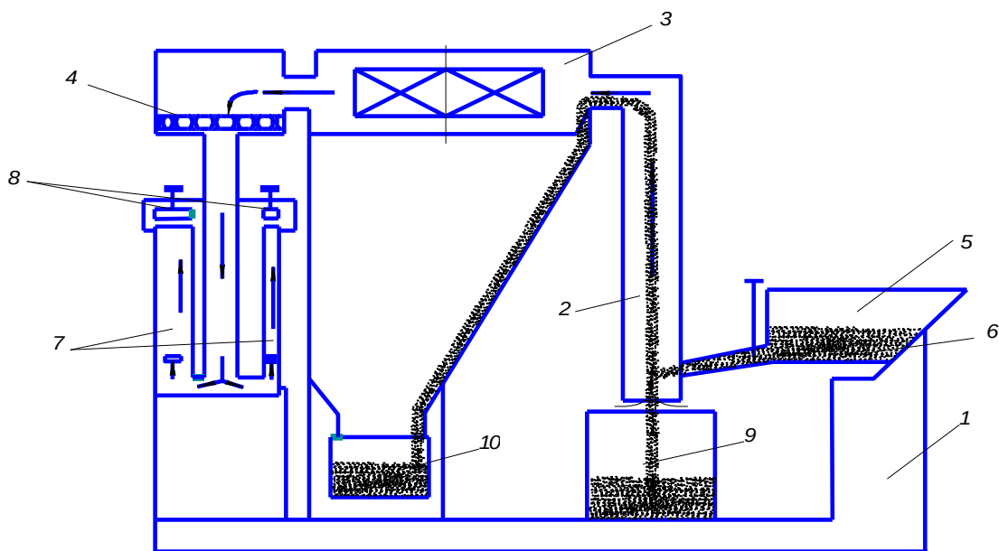
Рисунок 2. Схема лабораторной установки
