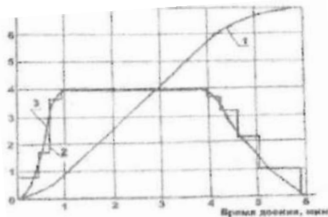
Рис. 6.4. Кривые надоя и потоков: 1 - кривая надоя; 2 - расчетный поток молока; 3 - реальный поток молока
