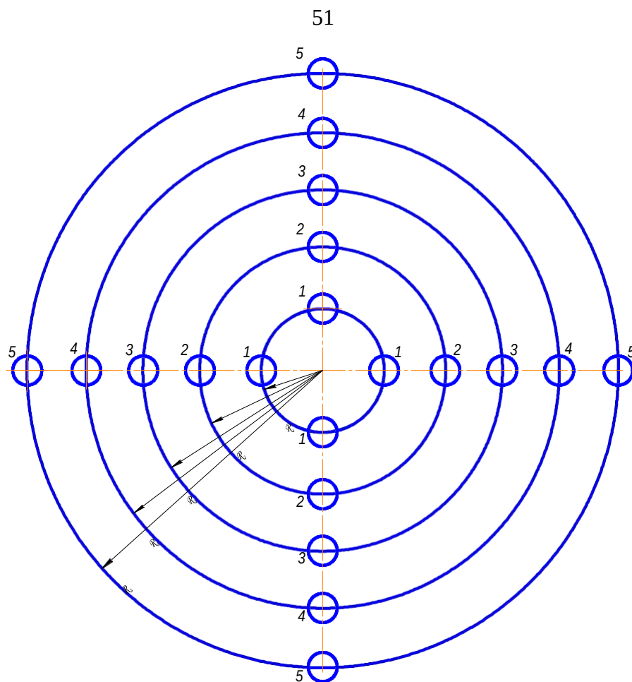
Рисунок 3. Порядок размещения дождемерных сосудов
