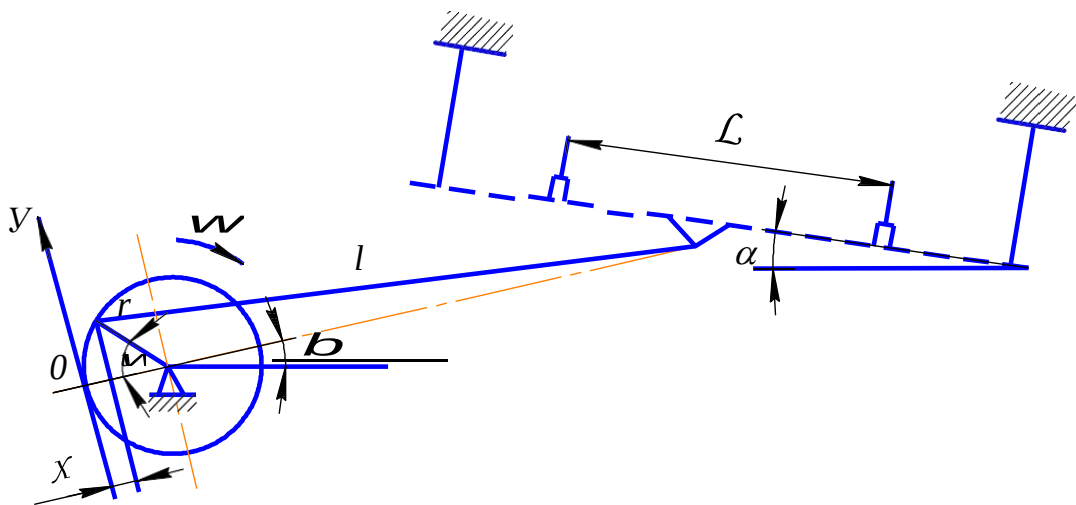
Рисунок 1. Схема работы решетного стана
