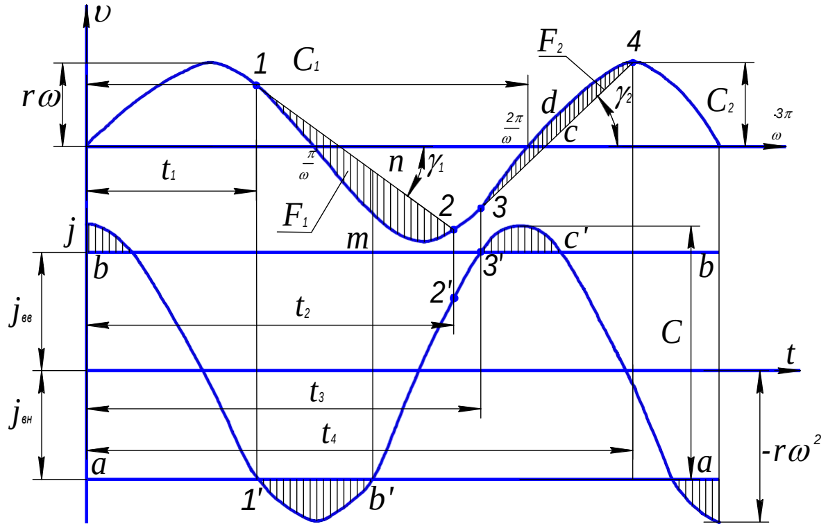
Рисунок 2. Графики скоростей и ускорений решетного стана и зернового материала
