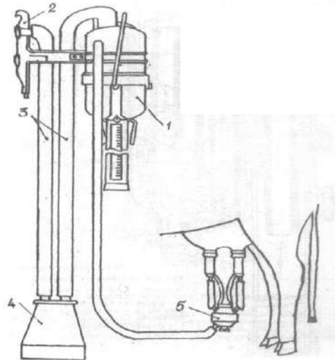
Рисунок 8.3. – Схема подключения УЗМ-1А на доильной установке с молокопроводом для определения погрешности измерения
