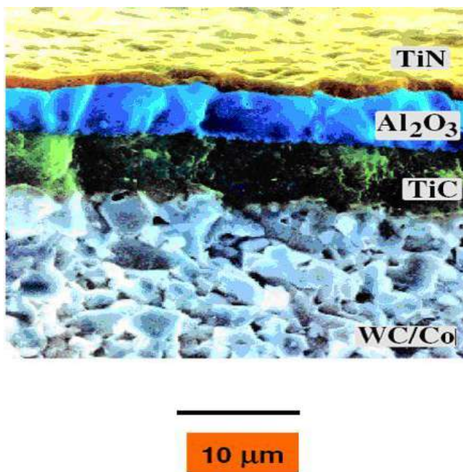
Рисунок 2 -Нанопокрyтия на подложке из WC/Co
