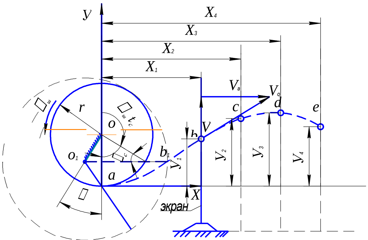
Рисунок 4. Схема к построению траектории движения частицы
