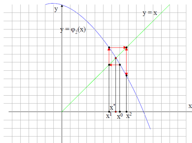
Расходящийся процесс простых итераций
