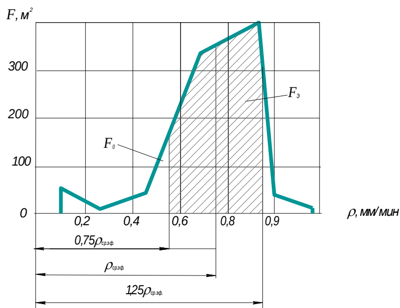
Рисунок 1. Зависимость размера площади от интенсивности полива
