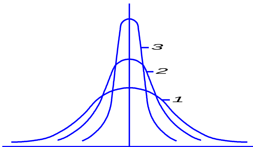
Рисунок 1. Кривые распределения с разными \sigma .
