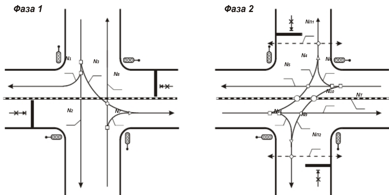
Рис. 13. Схема конфликтных точек на регулируемом перекрестке
