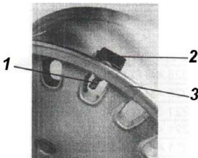
Рис. 2. Установка датчика-модуля на ободу колеса (внутренняя установка): 1 – вентиль (в качестве антенны); 2 – датчик-модуль; 3 – обод колеса
