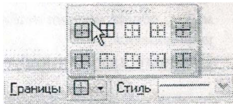
Рисунок 6.14. Выбор Границ .
