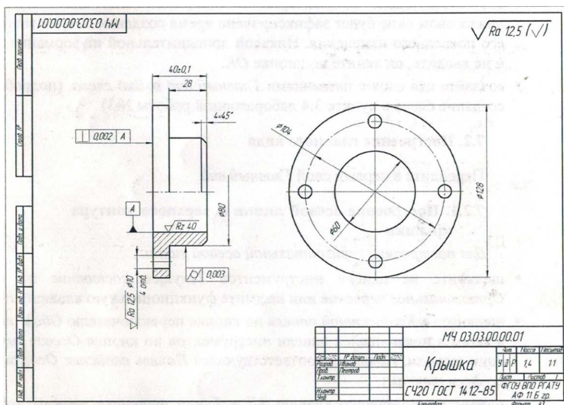
Рисунок 7.1. Крышка.
