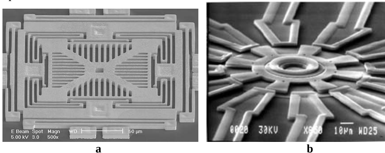
Рисунок 2. Изображение МЭМС-устройств, сделанное с помощью электронного микроскопа: а) трехосевой акселерометр; б) электростатический микродвигатель
