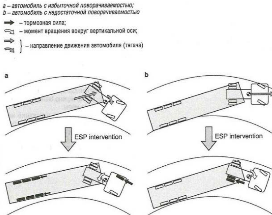
Рисунок 1 - Принцип тормозящего вмешательства ESP у полуприцепов» для ярко выраженной избыточной и недостаточной поворачиваемости, соответственно
