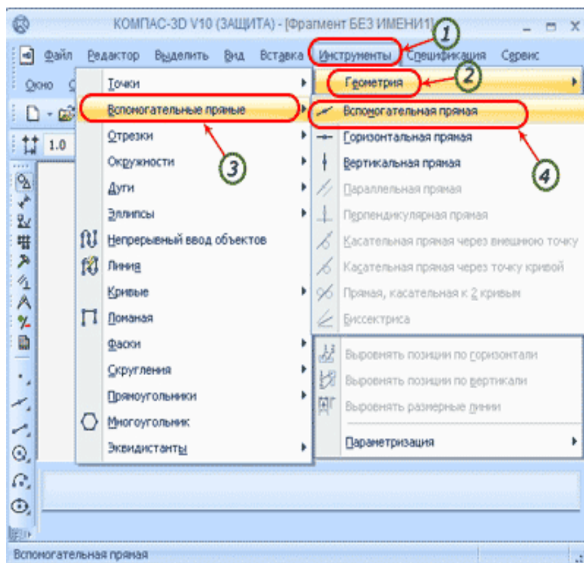
Рисунок 2.1 Панель геометрии.
