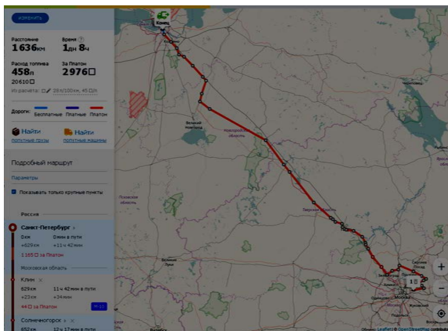
Рис. 7 Просмотр маршрута
