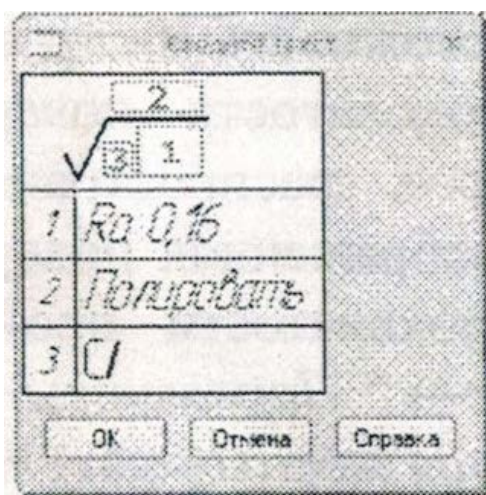
Рисунок 6.2. Диалог Текст
