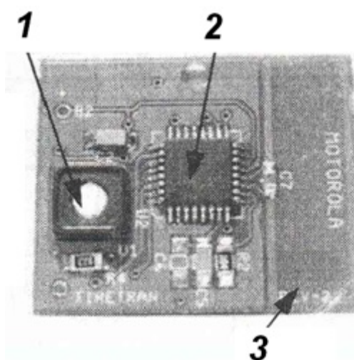
Рис. 6. Внешний вид демонстрационной платы модуля: 1 – датчик; 2 – кристалл микроконтроллера; 3 – рамочная антенна
