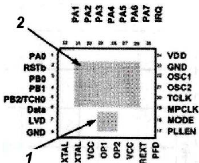
Рис. 4. Обобщенная структура микроконтроллера:
