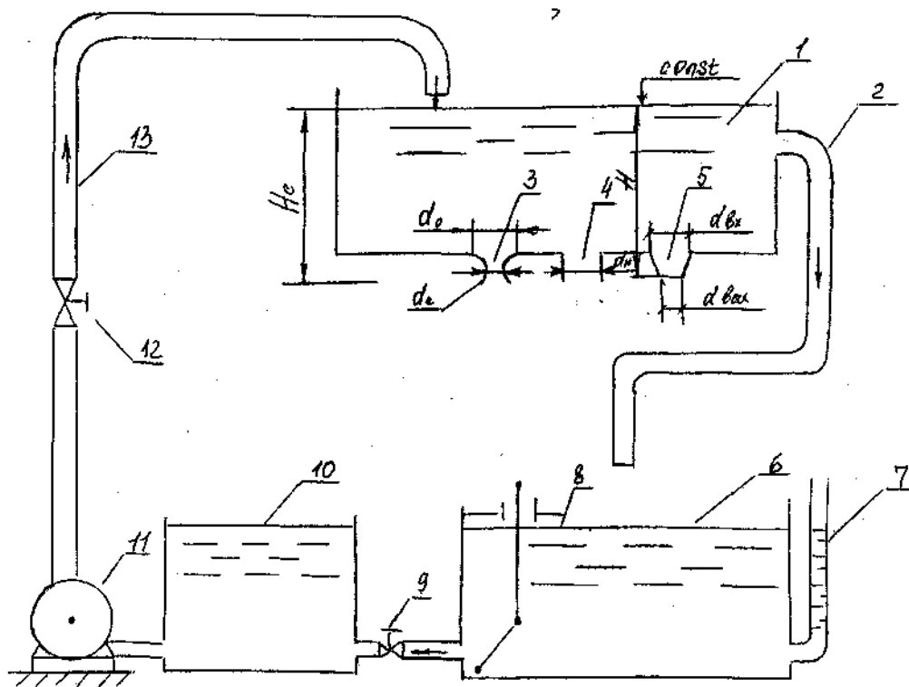
Рис. 7.6. Схема экспериментальной установки: 1 - напорный бак; 2 - слив; 3 - отверстие в тонкой стенке; 4 - цилиндрический насадок; 5 - конически сходящийся насадок; 6 - мерный бак; 7 - пьезометр; 8 - клапан; 9,12 - вентили; 10 - резервуар; 11 - насос; 13 - питающий трубопровод.
