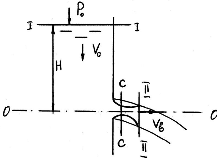
Рис. 7.5. Схема истечения из цилиндрического насадка.
