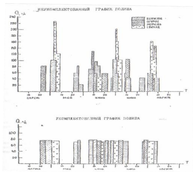
Рис.2 Графики полива
