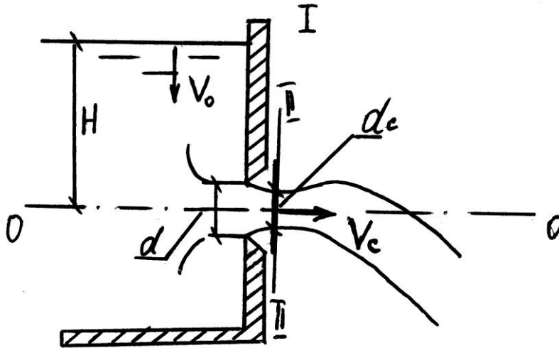
Рис. 7.3. Схема истечения из отверстия в тонкой стенке.
