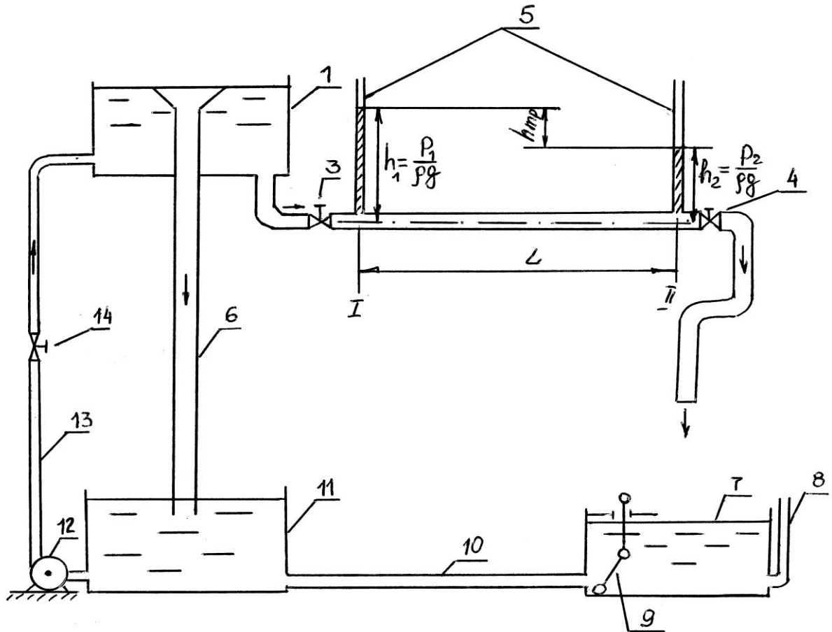
Рис. 5.2. Схема экспериментальной установки:
