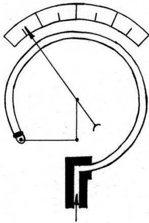
ПРУЖИННЫЙ МАНОМЕТР
