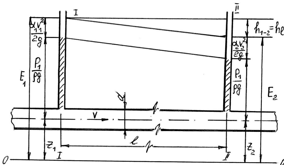
Рис. 5.1. Схема размещения контрольных створов и диаграммы уравнения Бернулли.
