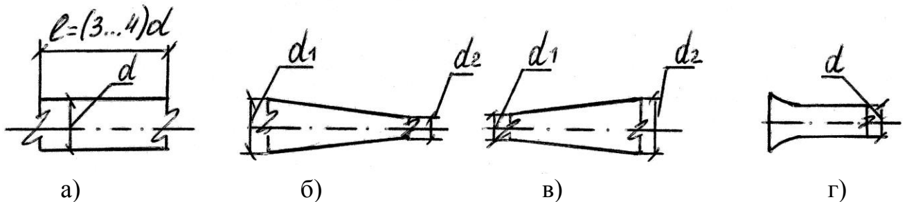
Рис. 7.4. Схемы насадков: а) цилиндрический; б) конически, сходящийся; в) конически расходящийся; г) коноидальный.
