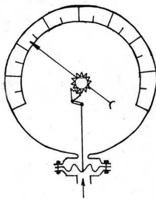
МЕМБРАННЫЙ МАНОМЕТР
