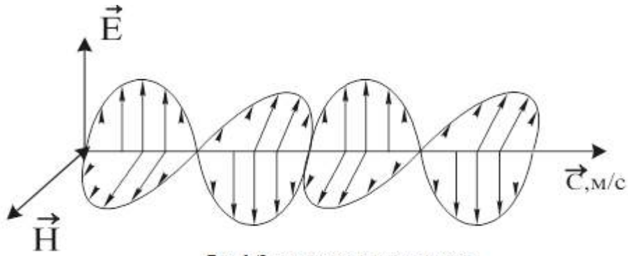
Рис.1 Электромагнитная волна
