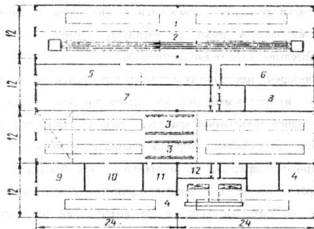
Рис. 7. 11. Компонировочный план вспомогательного корпуса АТП. 1-Пост общей диагностики; 2-Пост перестановки колес; 3-Поточные линии ЕО; 4-Малынная; 5-Склад шин; 6-Шинномонтажная; 7-Бытовые помещения; 8-Компрессорная; 9-Трансформаторная; 10-Такелажная; 11-Комната мойщиков; 12-Электрощитовая.
