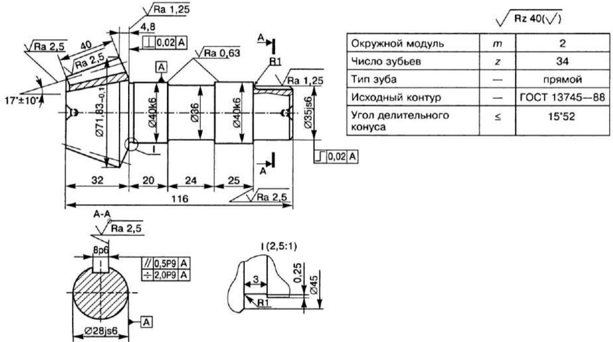
Рисунок 7 - Шестерня
