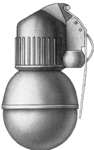
Наступательная граната РГН
