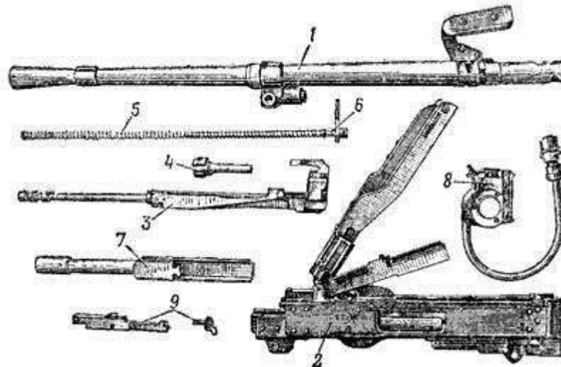
Основные части и механизмы пулемета ПКТ:
