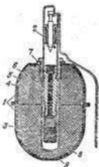
Граната РГД-5
