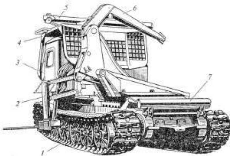
Рис. 3.1. Валочная машина ВМ-4:
