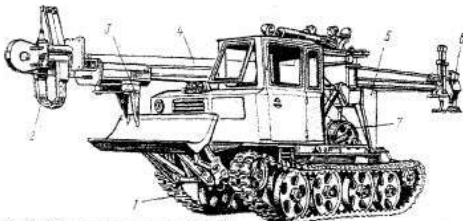
Рис. 62. Сучкорезная машина ЛП-30Г:
