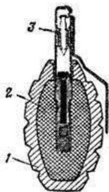
Граната Ф-1
