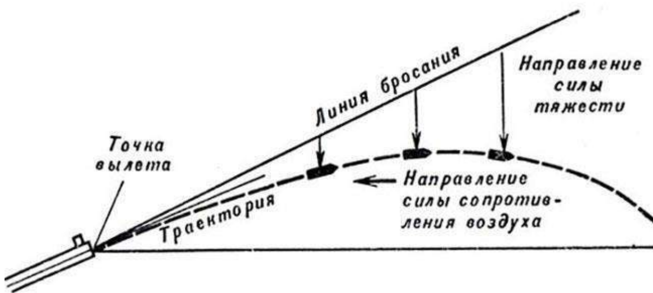
Рис. 60. Траектория полета пули
