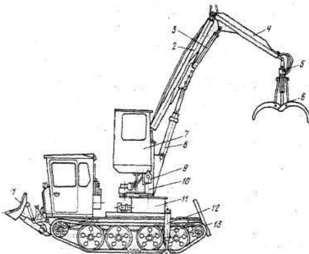
Рис. 4. Погрузчик-штабелер ПШ-80:
