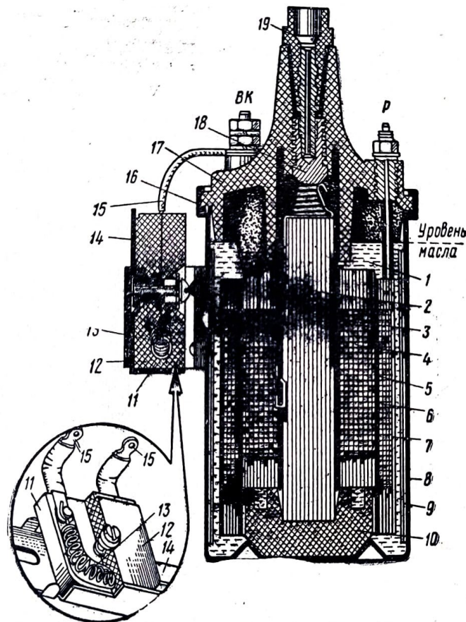
Рисунок 2 – Маслонаполненная катушка зажигания
