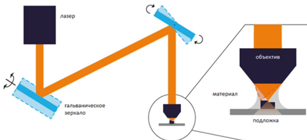
Рисунок 4 – Технология двухфотонной полимеризации
