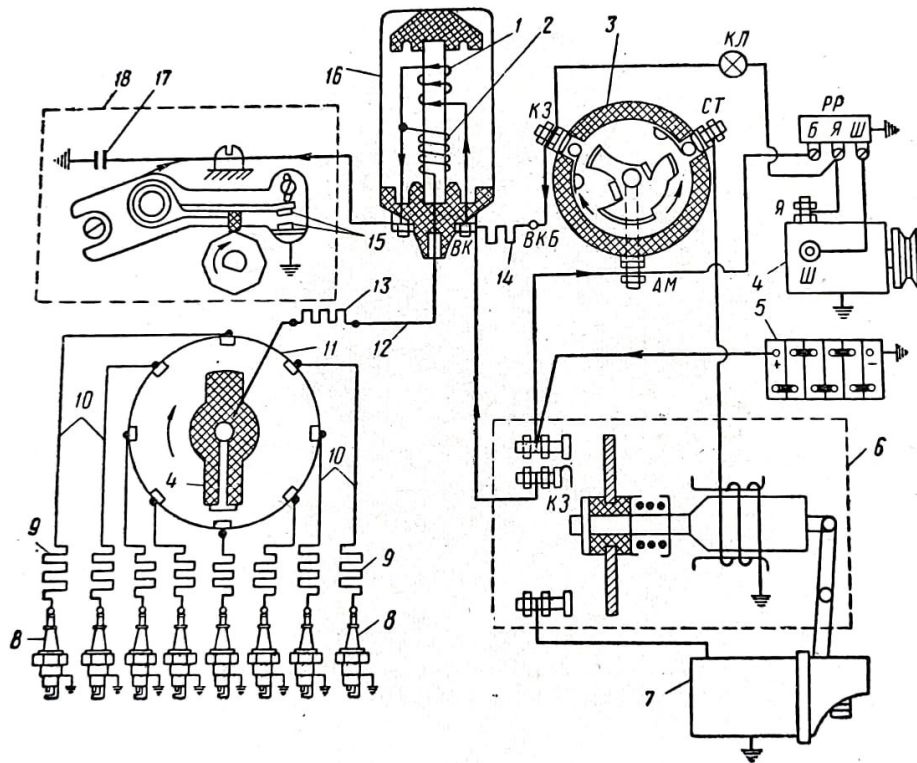
Рисунок 1 – Схема батарейного зажигания восьмицилиндрового двигателя
