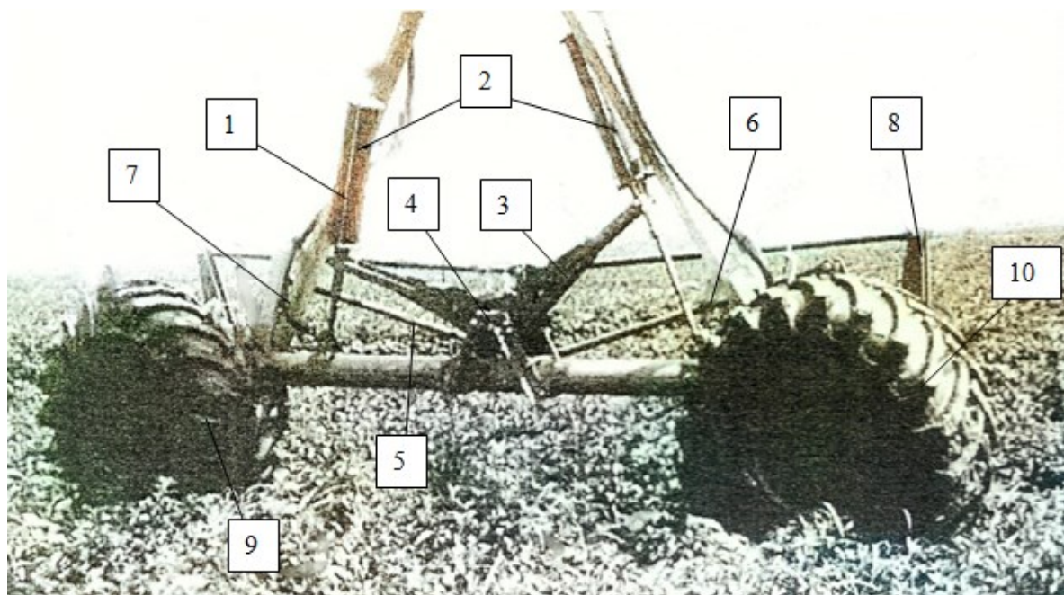
1 – рама; 2 – гидроцилиндр; 3 – большой двуплечий рычаг; 4 – меньший двуплечий рычаг; 5, 6 – тяга; 7, 8 – стопоры; 9 – приводное кольцо; 10 – пневмоколесо 21,3-24
