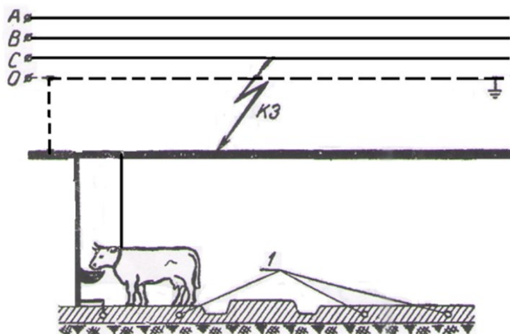
Рисунок 1 – Выравнивание распределения потенциалов внутри фермы: 1 – выравнивающие полосы; КЗ – место короткого замыкания
