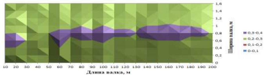
Рисунок 3 – Исследование профиля вала
