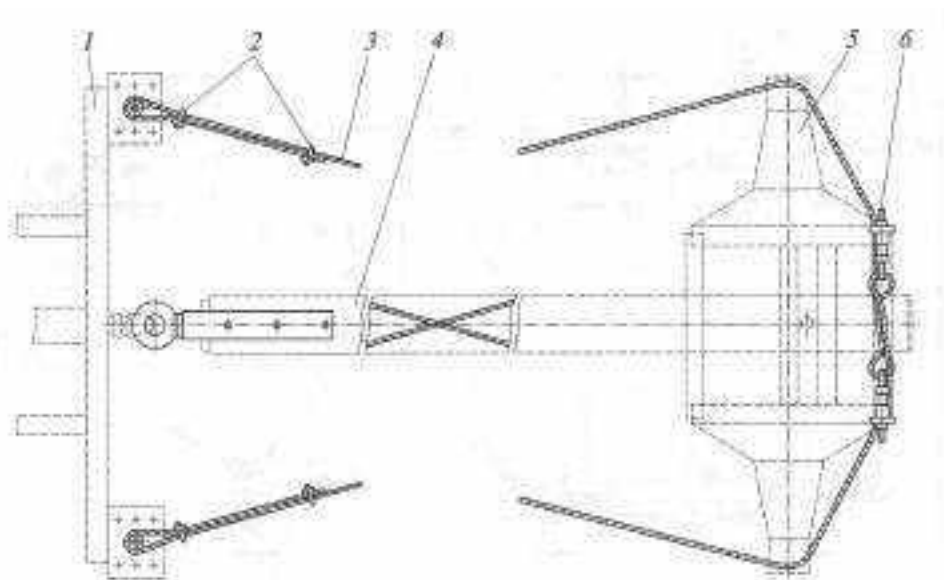
Рис. 4.3. Схема крестообразной сцепки: 1 — тяговая балка автомобиля; 2 — зажим; 3 — стальной канат; 4 — дышло; 5 — тяговая балка ропуска; 6 — рым-болт, регулирующий натяжение каната крестообразной сцепки
