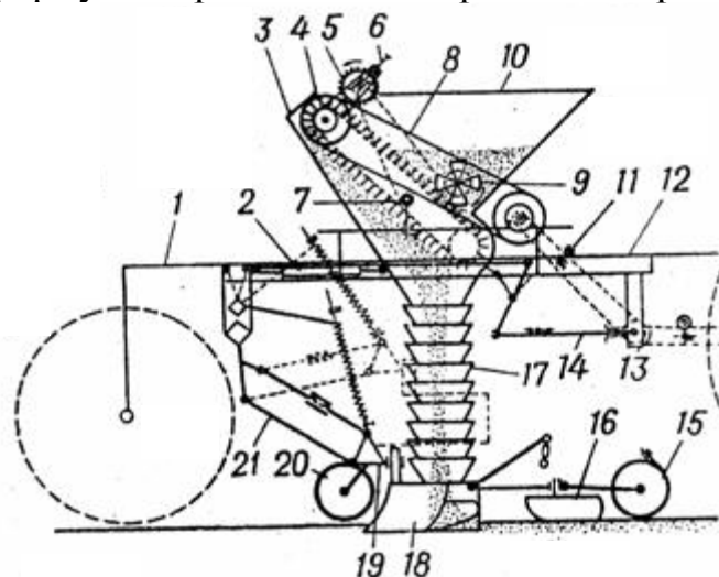
Рис. 12. Сеялка лесная питомниковая СЛПМ:
