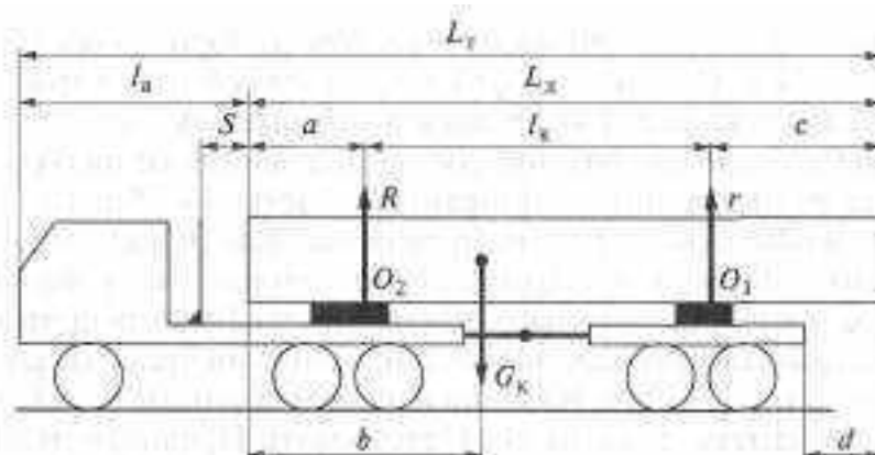
Рис. 4.4. Схема автопоезда к расчету расстояния между кониками: L_t — длина транспортного средства; L_x — длина деревьев или хлыстов; S — расстояние безопасности между пачкой хлыстов и защитной решеткой; c — расстояние от коника роспуска до крайней задней точки транспортного средства; d — свес груза
