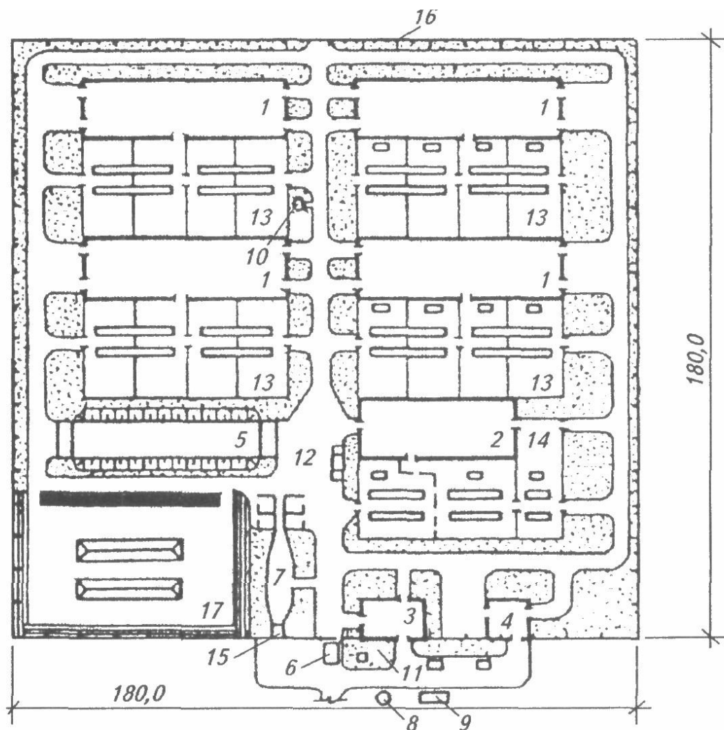
Генеральный план козоводческой фермы пухового направления на 3000 голов:
