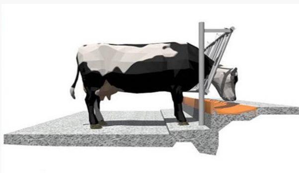
Рисунок 7 – Устройство кормового стола.
