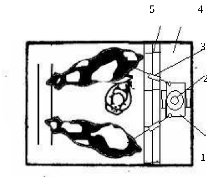
1 – мобильный модуль; 2 – емкость для сбора молока; 3 – пневмомеханический съемник доильных стаканов; 4 – навозный проход; 5 – навозная канавка
